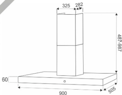
Рис. 1 Внешний вид кухонной вытяжки и схема размеров
